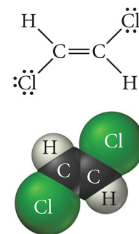
trans-1,2-dichloroéthène
