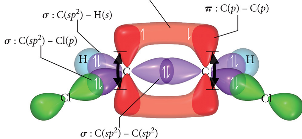
1,2-dichloroéthène
