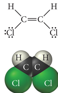
cis-1,2-dichloroéthène
